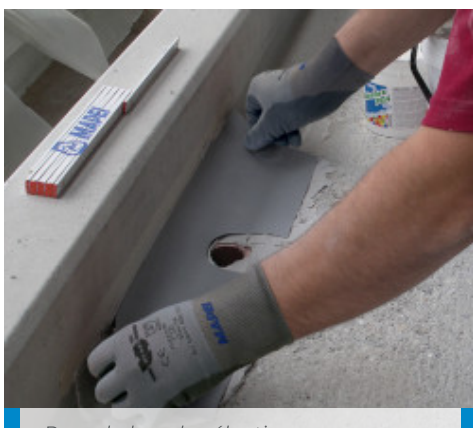
Pose de bandes élastiques en hypalon
