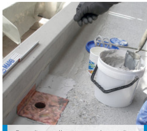
Pose d'une collerette en cuivre et d'un tuyau de drainage
